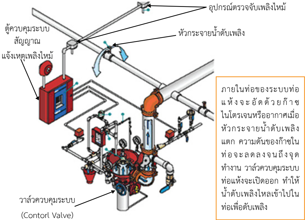
ภาพที่ ๓๑ การทำงานของระบบท่อแห้งแบบชลอน้ำเข้า (Pre-Action System)
