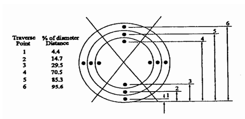
รูปที่ 7 แสดงการกำหนดจุดชักตัวอย่างตามลักษณะของปล่องที่เป็นปล่องวงกลม
