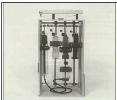
รูปที่ 10 แสดงเครื่องมือวิเคราะห์หาน้ำหนักโมเลกุลของอากาศด้วยเครื่อง Orsat analyzer
